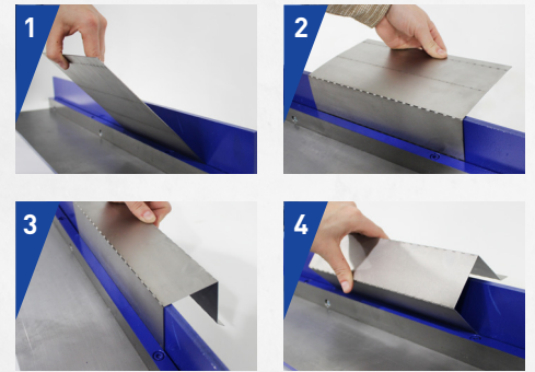
Biegereihenfolge für Schalungsblech
