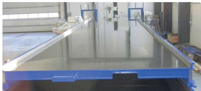
Após a renovação: superfícies de moldagem fechadas, retificadas e niveladas como novas; pintura totalmente revista e como nova
